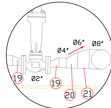
VISTA DETALLE B
