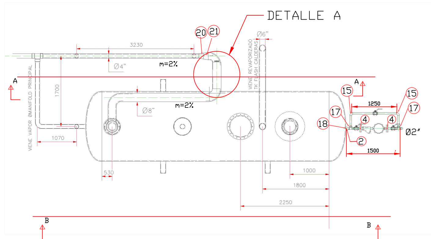
VISTA DE PLANTA
