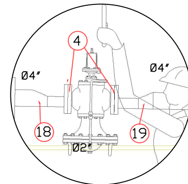
VISTA DETALLE C
